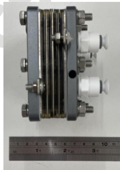
圖三:上視圖
